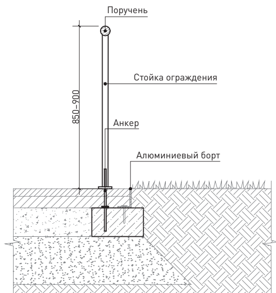
51 Схема установки пешеходного ограждения на эскалаторе
