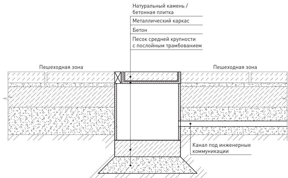
113 Схема устройства приемки подключения к подземным коммуникациям / сечение
